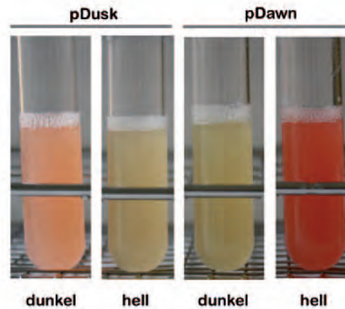
Abb 5: Das optogenetische System pDusk und das daraus abgeleitete pDawn vermitteln Lichtkontrolle über die Produktion beliebiger Proteine in bakteriellen Zellen. Wie hier beispielhaft für ein rot fluoreszierendes Protein gezeigt, sind die Unterschiede in der Produktion mit bloßem Auge erkennbar (Bild: Arbeitsgruppe Prof. Andreas Möglich).
