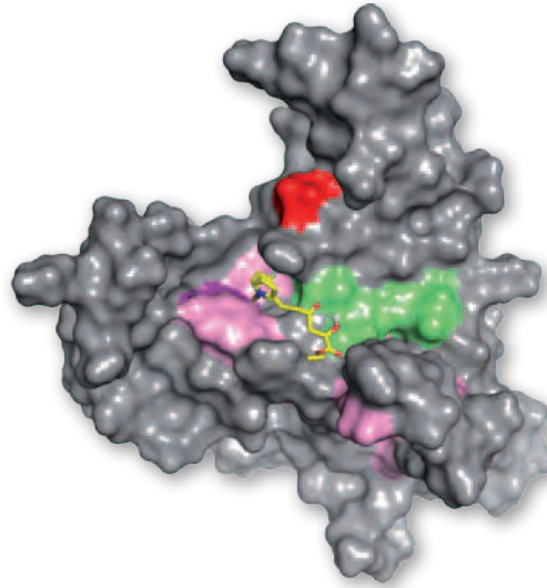
Abb. 4: Struktur der RNase H mit Inhibitmolekül RDS1643. Die dreidimensionale Struktur der RNase H ist grau, das aktive Zentrum der RNase H grün dargestellt. Die Aminosäuren, die durch die Inhibitorbindung beeinflusst werden, sind durch verschiedene Rotabstufungen markiert (Grafik: Anna Schneider-Fuchs).
