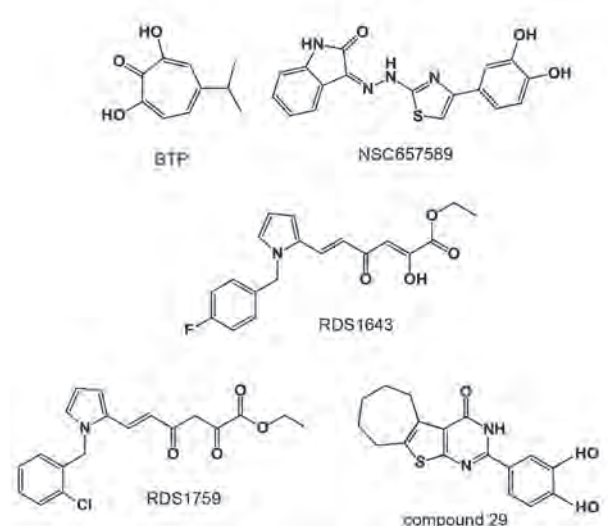
Abb. 3: Kleine Moleküle, die als RNase H-Inhibitoren wirksam sind. Der Inhibitor RDS 1643 wurde für die NMR-spektroskopischen Untersuchungen an der Universität Bayreuth verwendet.
