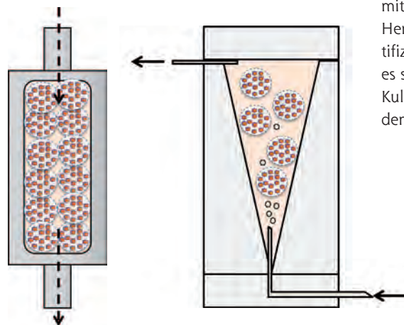
Abb. 6: Im Festbettreaktor (li.) können sich die Kapseln mit den darin eingeschlossenen T-Lymphozyten nicht bewegen und werden von einer Nährflüssigkeit durchströmt; im Wirbelschichtreaktor (re.) werden sie von der Nährflüssigkeit in ständiger Bewegung gehalten (Grafiken: Dr. Valérie Jérôme).
