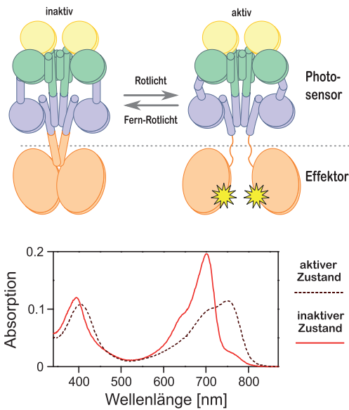
Abb 4: Die künstlich erzeugte Phosphodiesterase LAPD vermittelt den Abbau wichtiger biologischer Botenstoffe. Die Absorption von Rotlicht löst weitreichende Strukturveränderungen aus, die eine erhöhte enzymatische Aktivität bewirken. Durch Bestrahlung mit Licht im Fern-Rot Bereich kann das Protein wieder inaktiviert werden. Auch im Absorptionsspektrum sind die Unterschiede zwischen aktivem und inaktivem Zustand zu erkennen (Bild: Arbeitsgruppe Prof. Andreas Möglich).
