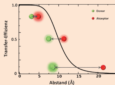
Abb. 5: Abstandsabhängigkeit der Energietransfereffizienz eines grünen Fluoreszenzdonors auf einen roten Fluoreszenzakzeptor (Förster-Radius 10 Å). Wenn beide Moleküle sehr nah beieinander sind, sieht man nur die Fluoreszenz des roten Akzeptors. Je weiter sich die beiden Moleküle voneinander entfernen, desto schwächer wird die Fluoreszenz des Akzeptors und desto intensiver wird die Fluoreszenz des Donors (Grafik: Elisa Bombarda).
