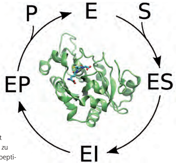
Abb. 1: Schematische Darstellung eines enzymatischen katalytischen Zyklus. Ein Substratmolekül (S) bindet an ein Enzym (E) und bildet einen Enzym-Substrat-Komplex (ES). Das Enzym modifiziert das Substrat meist über einen oder mehrere Intermediate (I) zum Produkt (P), das schließlich vom Enzym dissoziiert. Das Enzym ist dann frei für einen neuen katalytischen Zyklus (Grafik: Elisa Bombarda).
